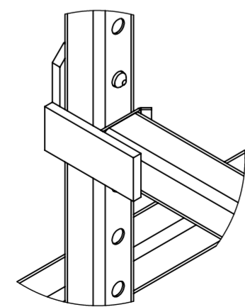
DETTAGLIO A SCALA 1 : 5
