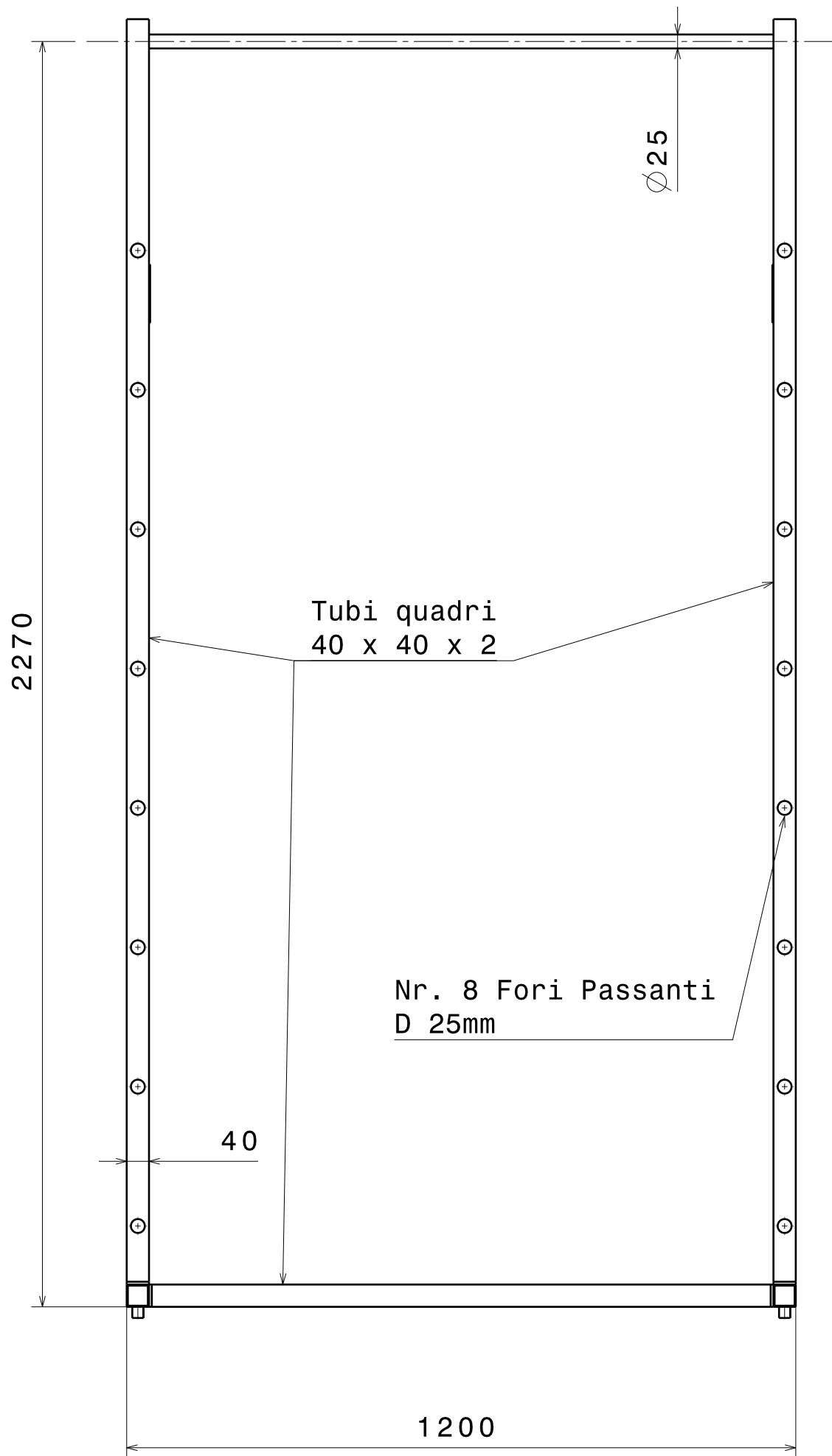
Vista frontale Scala: 1:10
